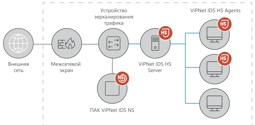
Рисунок 1. Схема подключения в физической сети
