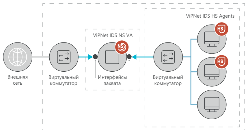
Рисунок 2. Схема подключения в виртуальной сети
